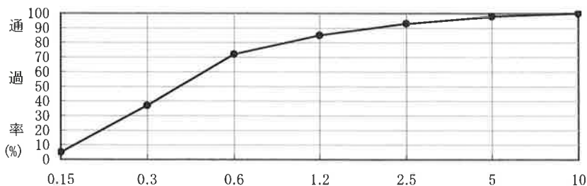
粒度曲線
